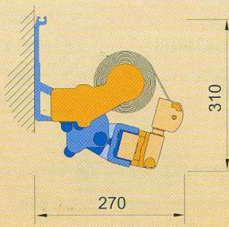
Montáž do stěny
