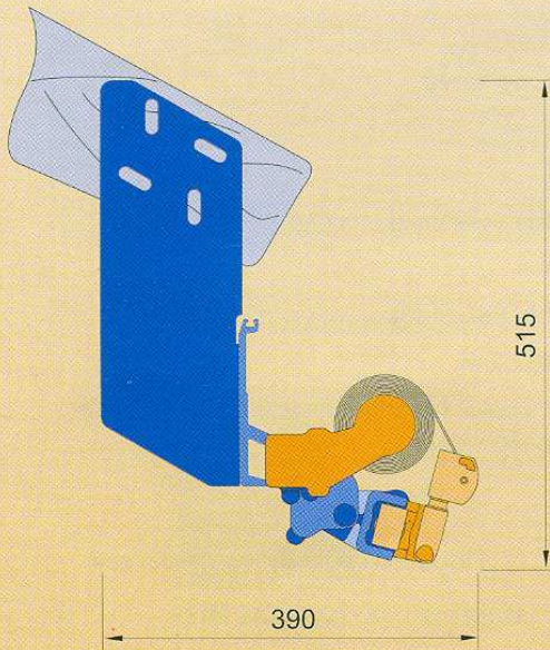
Montáž do krovu
